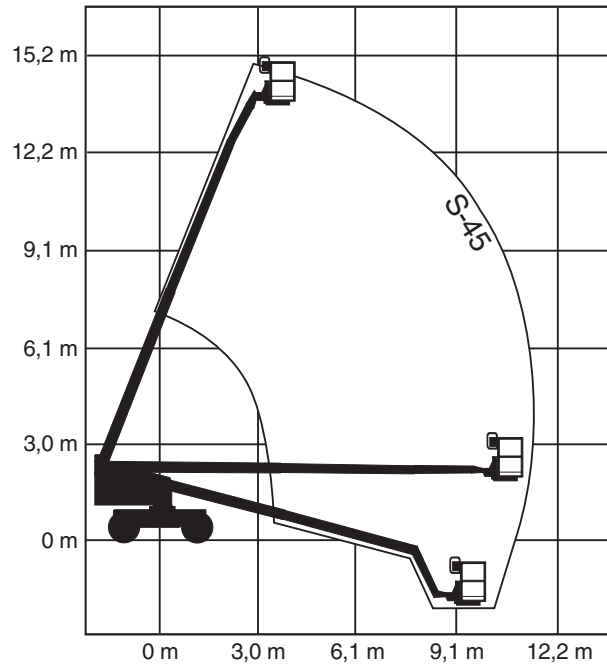
S-45 Diagram over bevegelsesområde
